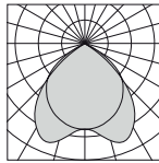
Doble parabólico Parabolic double
