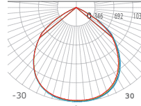
Prismático UGR<19 Prismatic UGR<19
